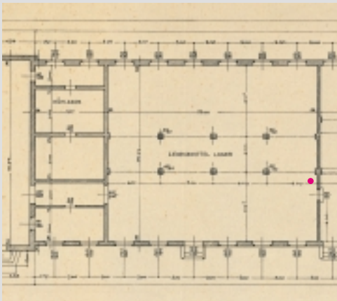
2001 ⑩ Grundrissplan des Wirtschaftsgebäudes, Maßstab 1 : 100, gefertigt von der Zentralbauleitung der Waffen-SS und Polizei, München-Dachau, 26. Februar 1944 (Ausschnitt: Lebensmittellager) Bayerische Hauptstaatsarchiv, München Ground plan of the maintenance building, scale 1 : 100, made by the Building Site Supervision Office of the Waffen-SS and Police, Munich-Dachau, February 26, 1944 (detail: Food storeroom)
